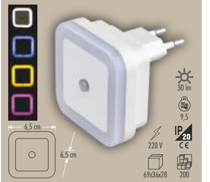
CT-9500 FOTOSELLİ GECE LAMBASI
