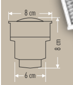
CT-9188 MİNİ SENSÖR
