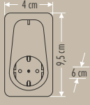
CT-9180 MEKANİK ZAMAN SAATİ
