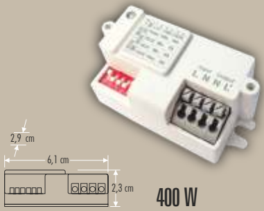
CT-9184 W OTOMAT ZAMAN SAATİ
