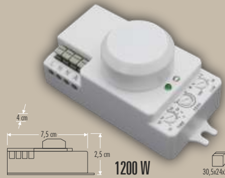
CT-9185 RADAR SENSÖR
