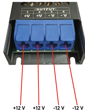
BAĞLANTI ŞEMASI/ CONNECTION DIAGRAM
